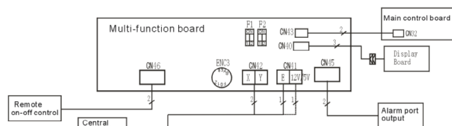
Schéma de connexion Multi-function board
